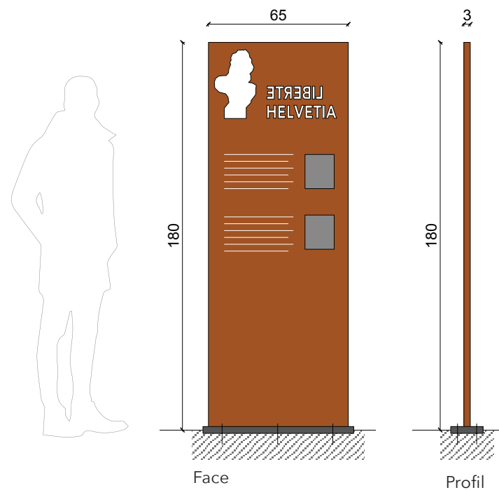
Panneaux verticaux avec perforations, 1:25
